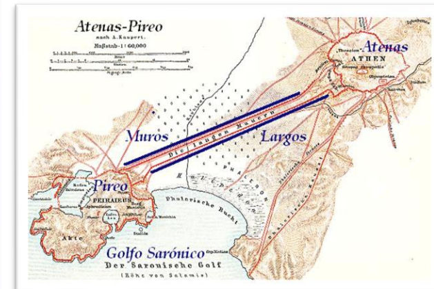
Mapa del puerto del Pireo y de los "muros largos" que unían el puerto con la ciudad de Atenas en el siglo V a.C.
